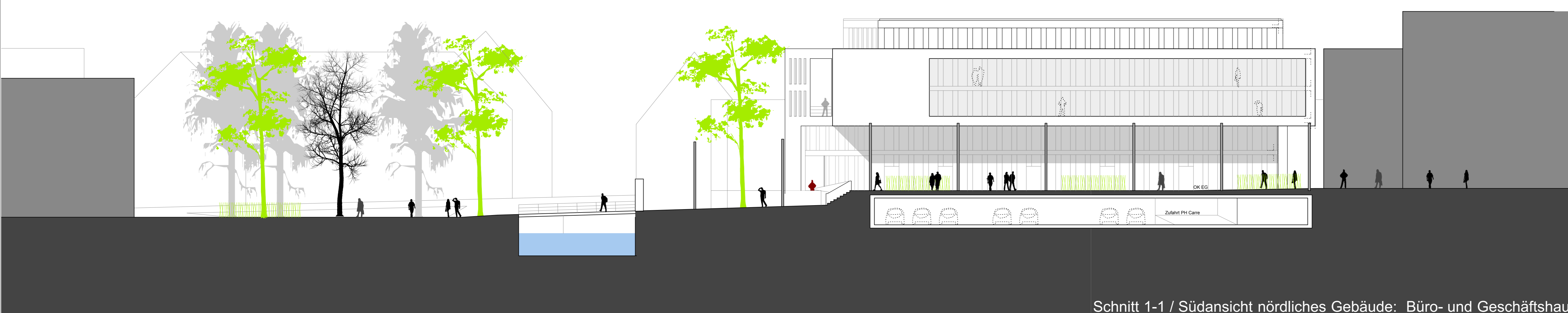
Schnitt 1-1 / Südansicht nördliches Gebäude: Büro- und Geschäftshaus
